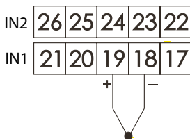
thermocouples
