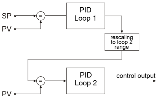
Fig. 24. Cascade control
