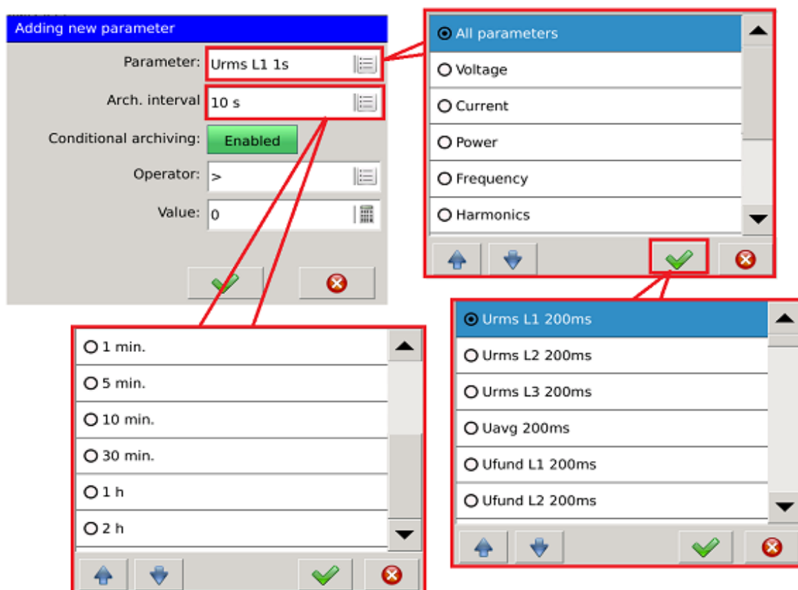
Fig. 124. Archiving – new parameter.
