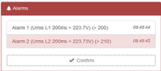
Fig. 83. Web server - alarm 2.
