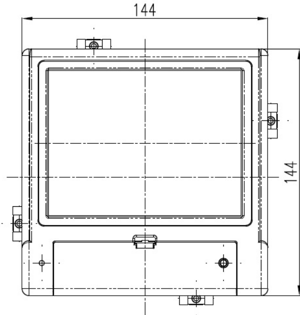
Fig. 13. Dimensions - front.
