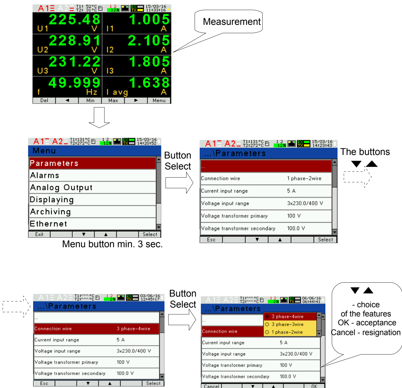
Fig. 15. Screens of Parameters mode
