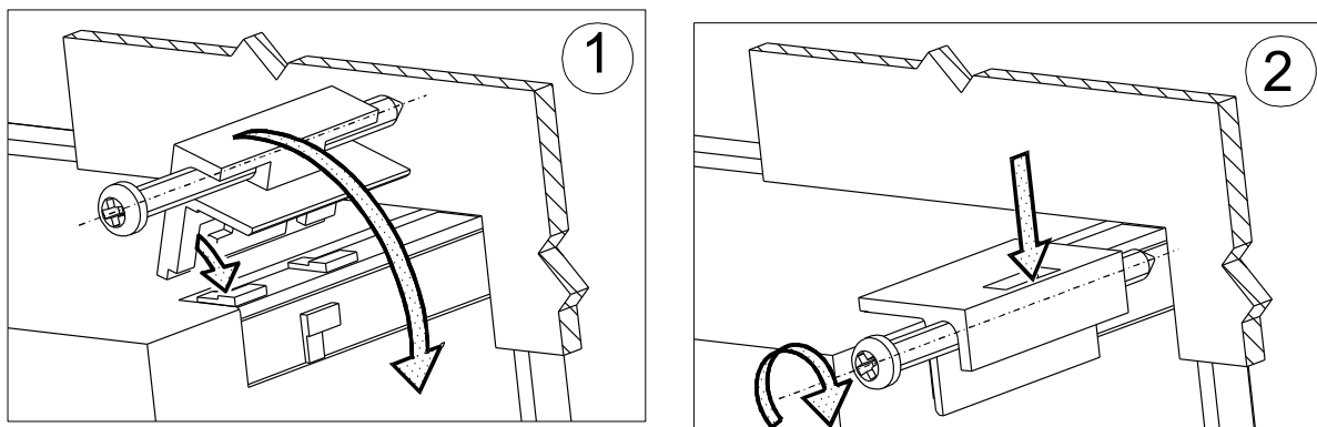
Fig. 2. Meter fitting
