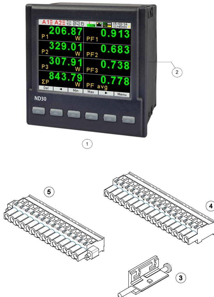
Fig. 1. Meter set
